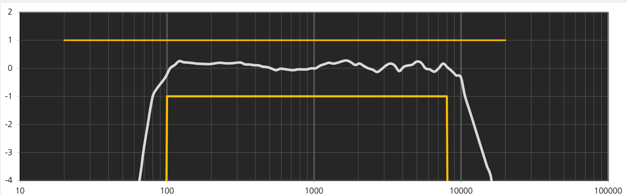
TalkBox 典型频率响应
